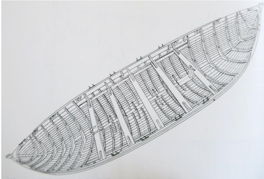
Teikning af Agli í Íslenskum sjávarhátum II.
