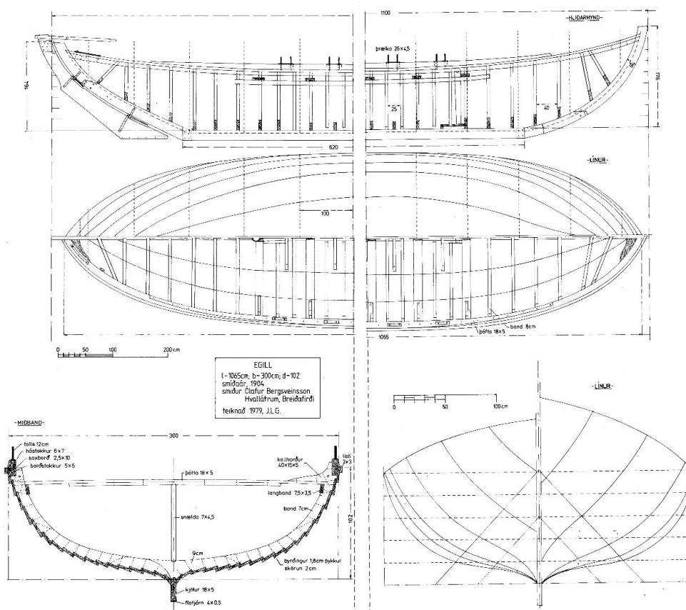
Teikning af bátnum Agli í Íslenskum sjávarhátum eftir Lúðvík Kristjánsson: Teikning: JLG 18
